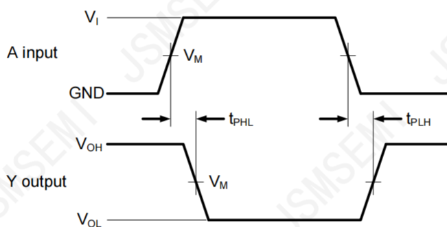
图5 输入A到输出Y的输延迟及输出转换时间
