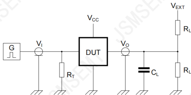
图4 测试开关时间的测试电路
