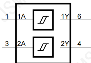
图1 逻辑符号
