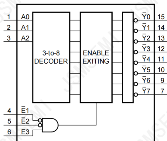
图 2 功能框图
