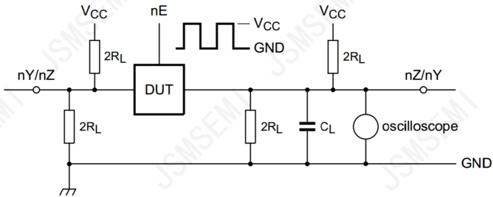
a. Circuit
