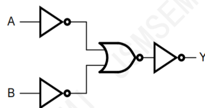
图 3 逻辑框图
