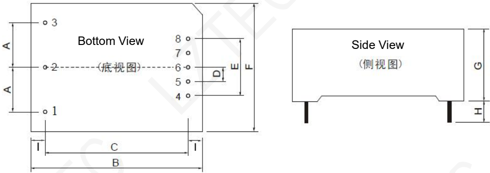
外壳尺寸 Shell Size (单位: mm)
