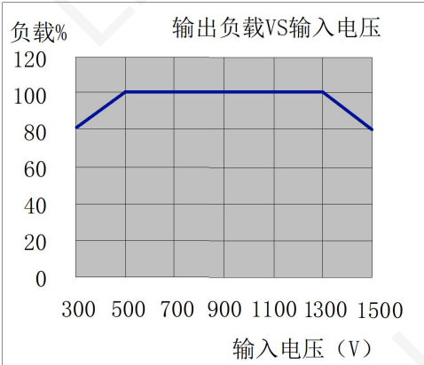
输出负载 Vs 输入电压曲线图 Output Load vs. Input Voltage Curve
