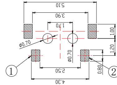
PCB. 焊接图
