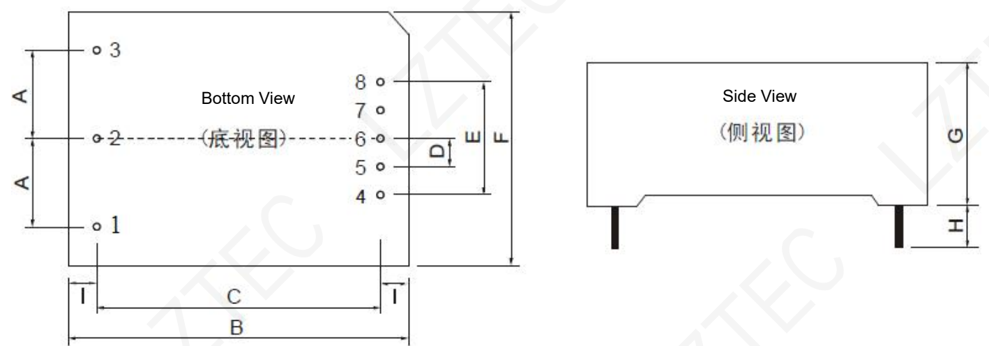
外壳尺寸 Shell Size (单位: mm)
