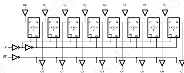
图 4 逻辑框图
