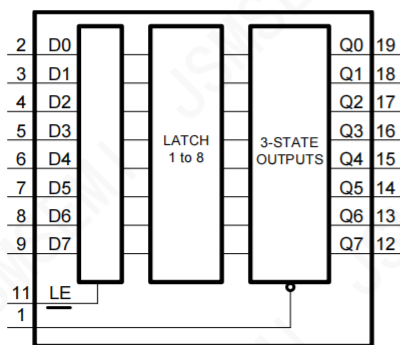
图 3 功能框图
