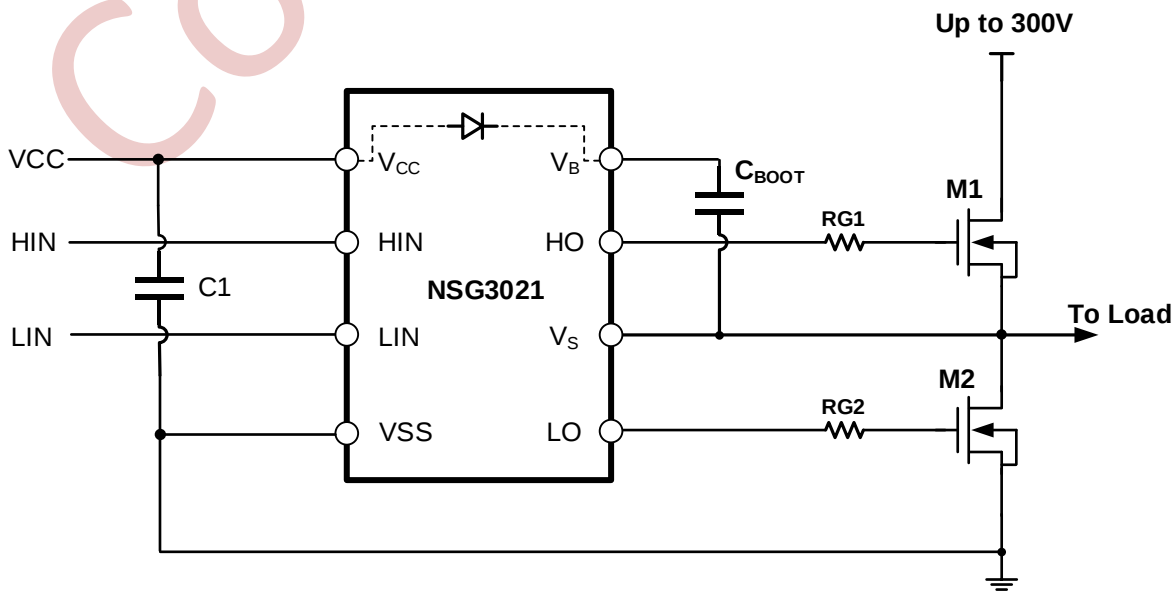
图 10-2 NSG3021 典型应用电路图
