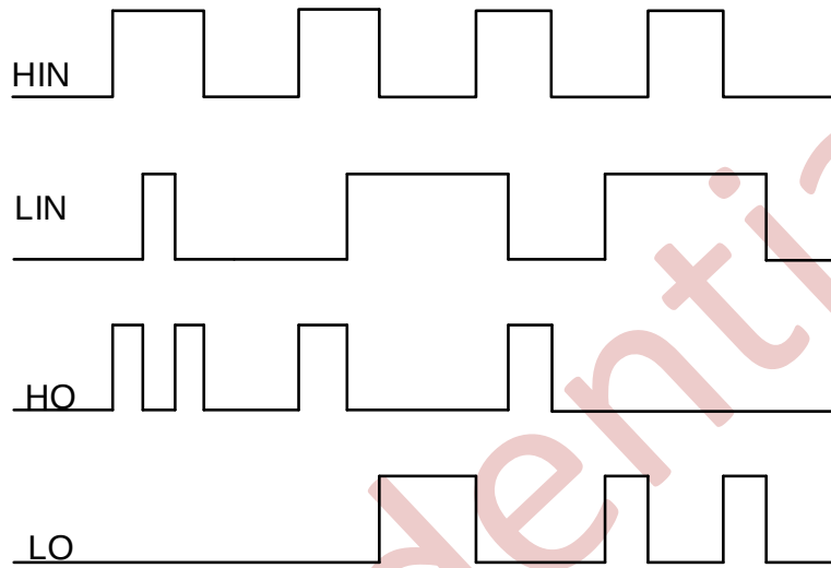
图 9-1 NSG3021 输入输出时序波形
