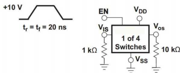
图 2 串扰控制输入到输出
