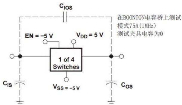
图 5 电容测试电路
