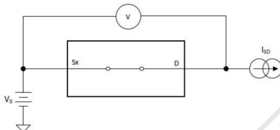
图 1 RON 测试
