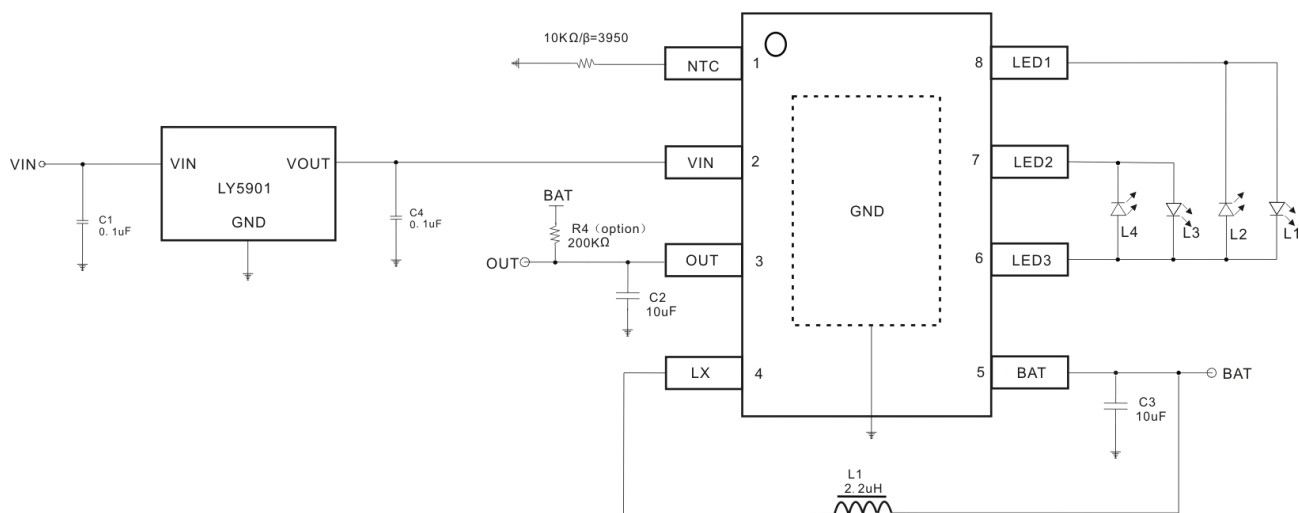
Fig2.带 OVP 应用电路
