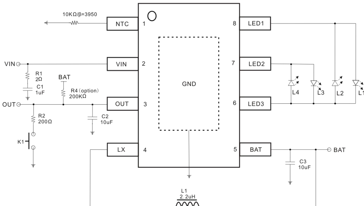
Fig1.LY6294TD 典型应用电路
