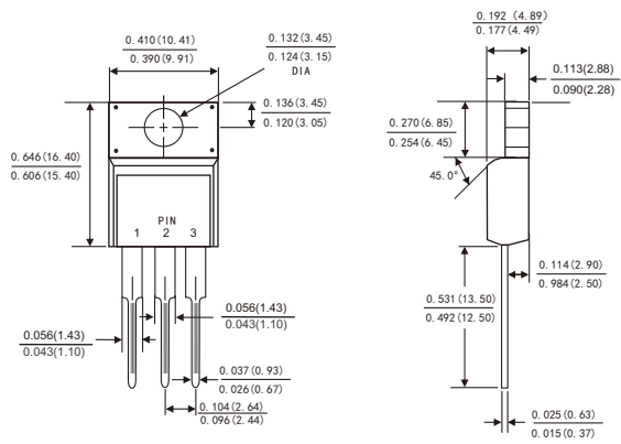
ITO-220AB
