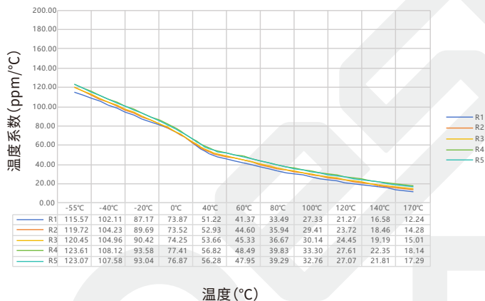
PEWM 3920系列 0.5mΩ温度系数实测数据表
