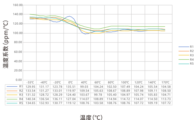
PEWM 3920系列 0.2mΩ温度系数实测数据表
