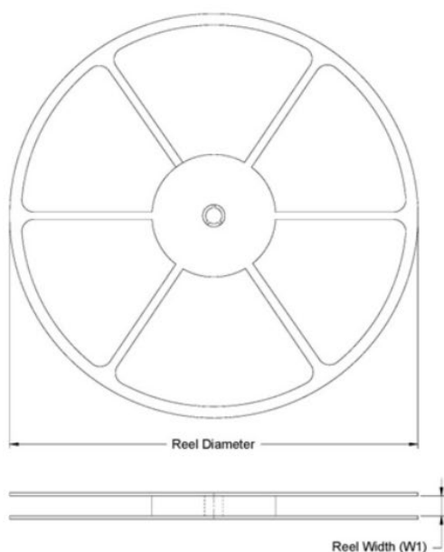
REEL DIMENSIONS
