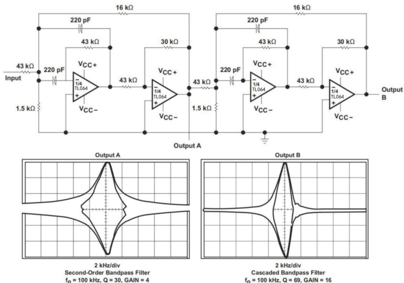
图1 正反馈带通滤波器
