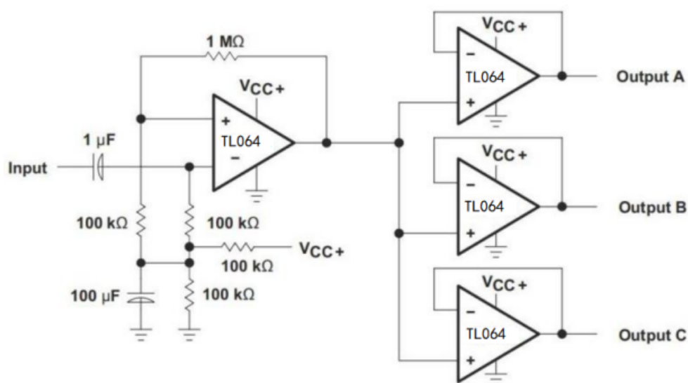
图2 音频分配放大器
