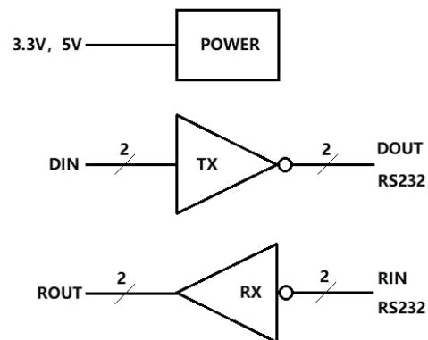
图2: HGX3232A 逻辑图
