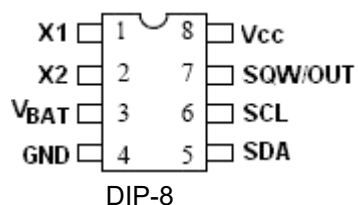
DIP-8
