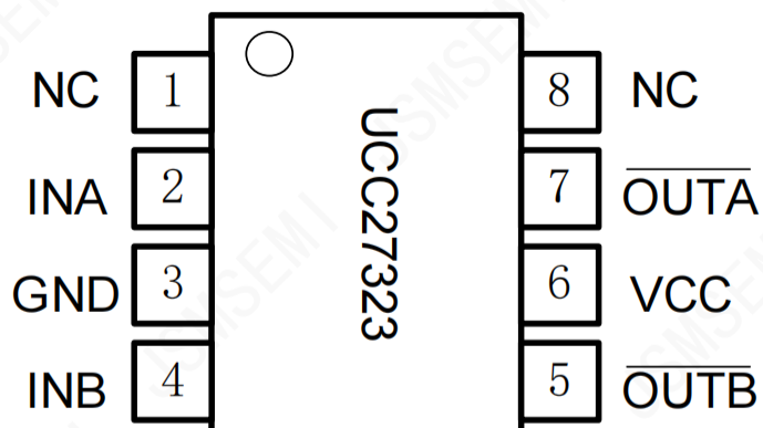
芯片引脚描述
