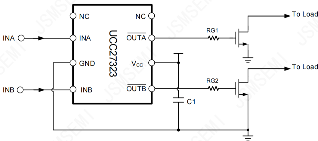
图 8-1 UCC27323 典型应用电路图
