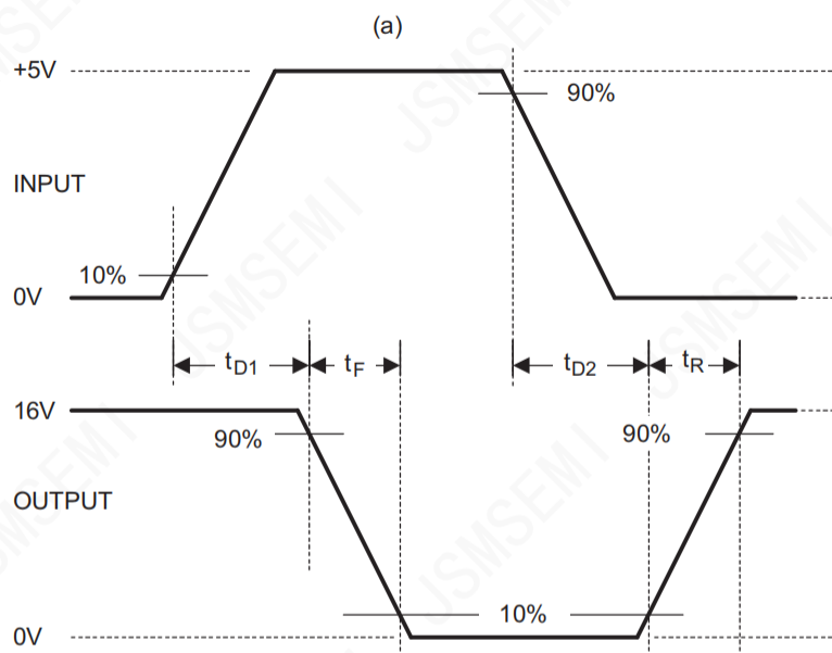
图 6-1 输入输出(反相)波形图
