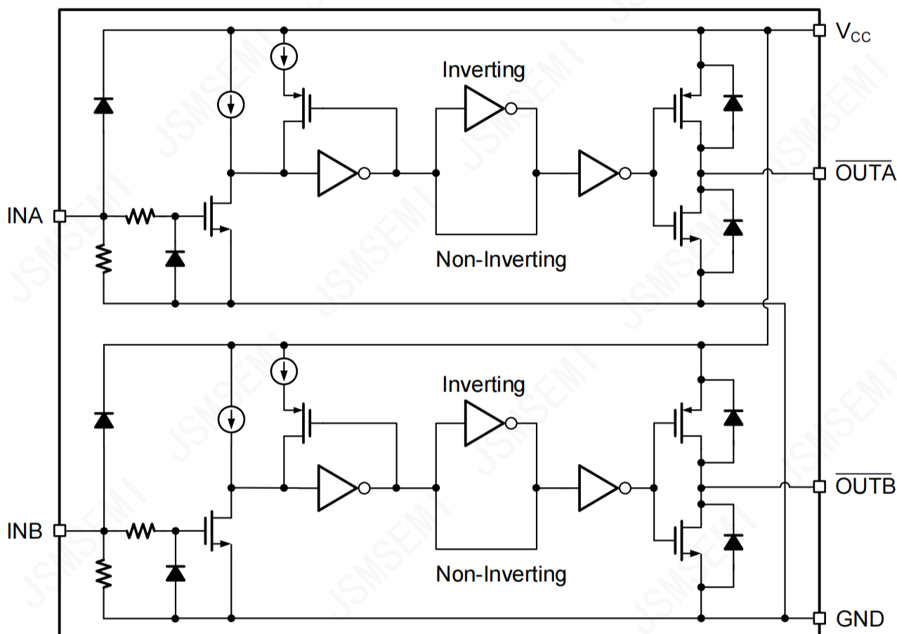
图 7-1 UCC27323功能框图
