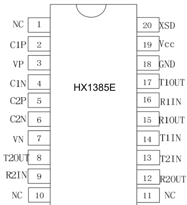
20-pin SSOP/TSSOP
