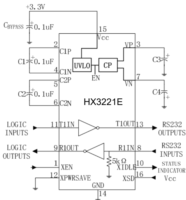
16-pin SSOP/TSSOP
