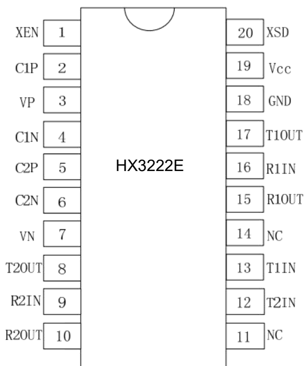
20-pin SSOP/TSSOP
