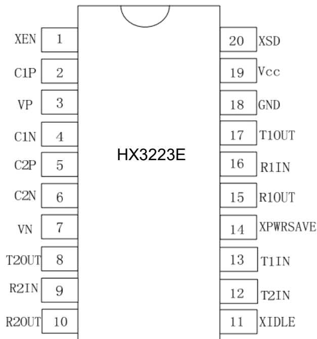
20-pin SSOP/TSSOP
