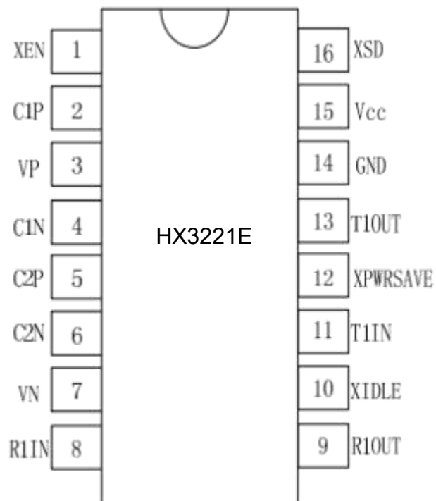
16-pin SSOP/TSSOP
