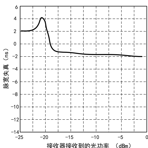
图 2 在 5MBd 速率下 NRS15x8Z/25x8Z 的脉宽失真
