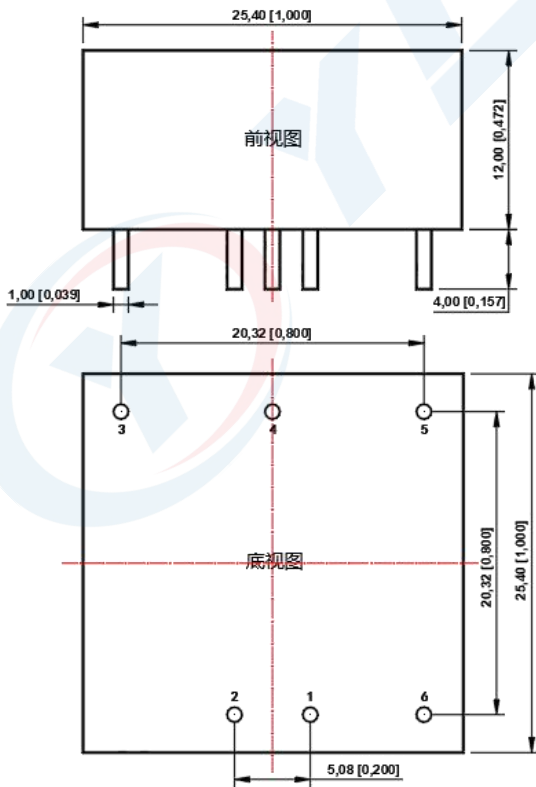
外观尺寸图
