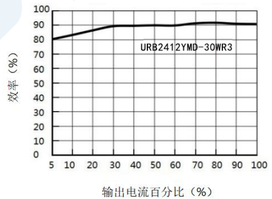
效率 VS 输出负载曲线图 (Vin=48V)
