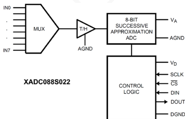
原理图
