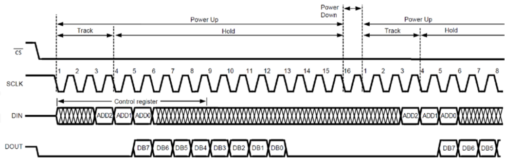
XADC088S022 操作时序图
