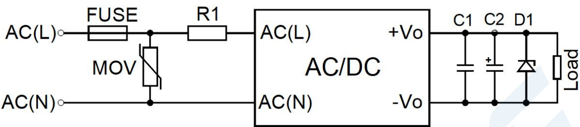
EMC 推荐电路（2-1）
