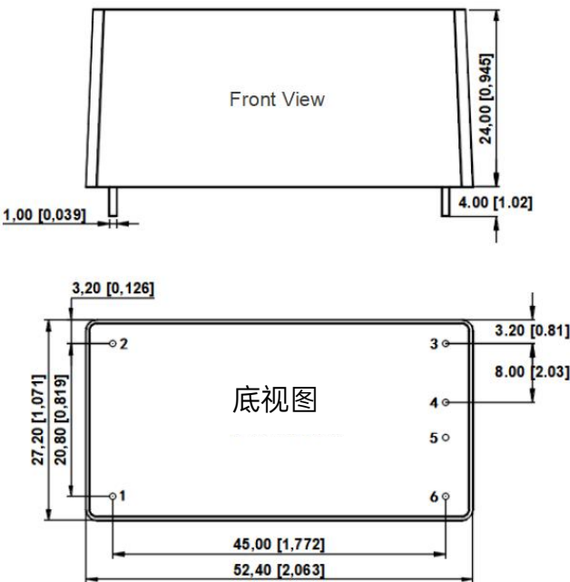
LD20-23BxxR2 外观尺寸图
