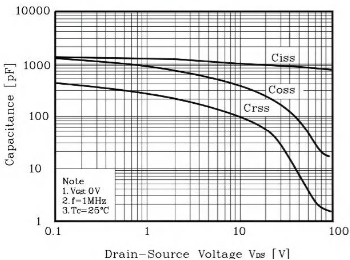
Fig. 5 Capacitance - V_{DS}
