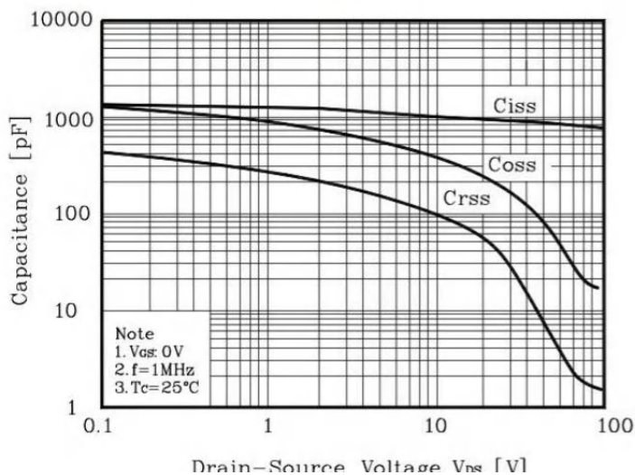
Fig. 5 Capacitance - V_{DS}
