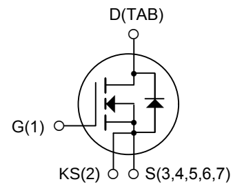
TO-263-7L
