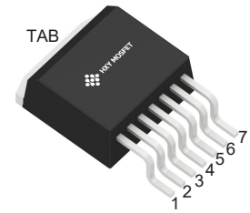
TO-263-7L
