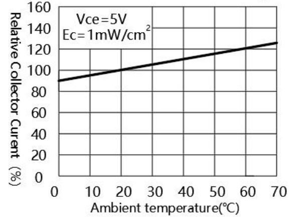
相对集电极电流与环境温度的关系 Relative Collector Current VS Ambient Temperature
