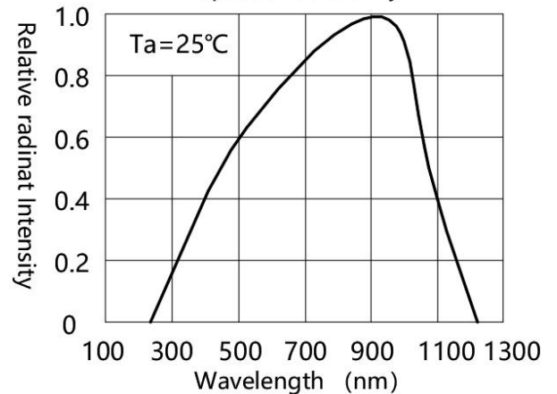
感应波长曲线图 Spectral Sensitivity
