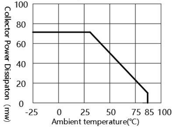
集电极功率与环境温度的关系 Collector Power Dissipation VS Ambient Temperature
