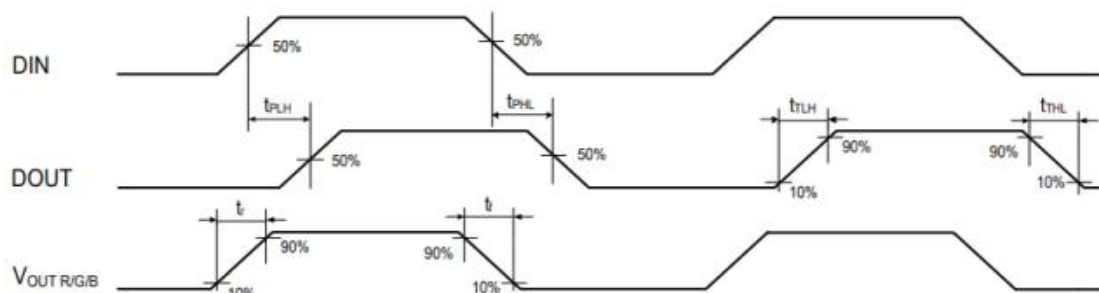
Fig.动态参数测试示意图
