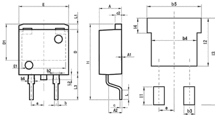
TO-263L, [-], (TO-263L)
