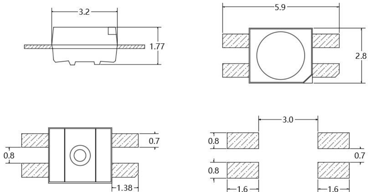
建议焊盘尺寸
