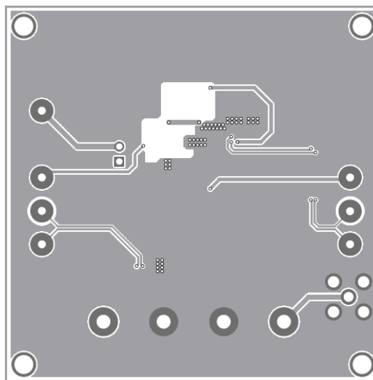
Bottom Layer
