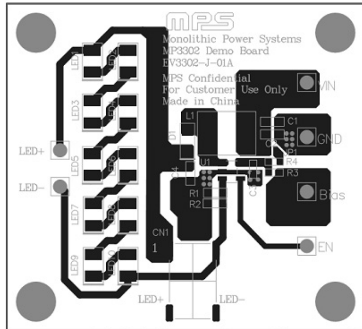
Figure 1—Top Layer
