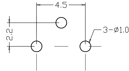
PCB线路板图
