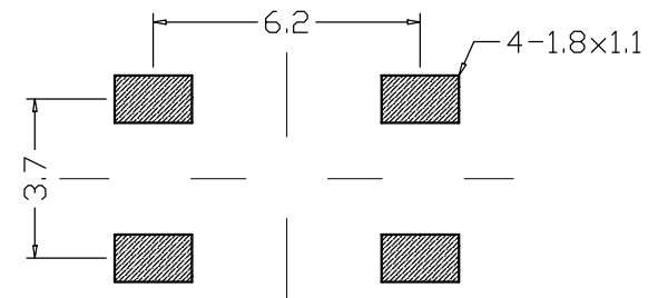
PCB线路板图
