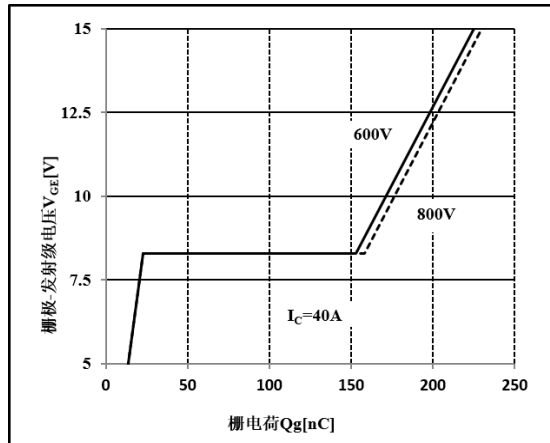
图 18 栅电荷特性
