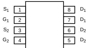
MSOP8
