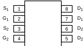
MSOP8
