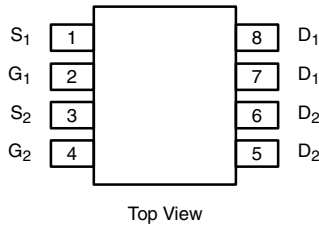
MSOP8
