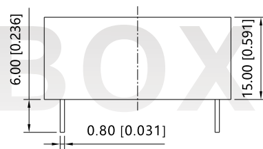
前视图
