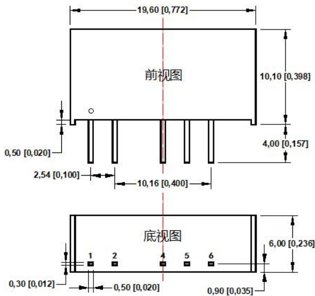
外观尺寸图
