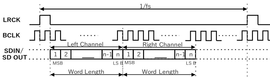
DSP_A mode (Offset=1)
