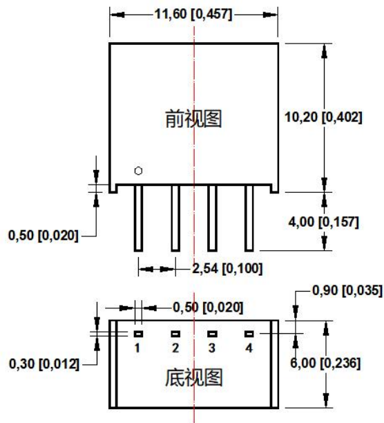
外观尺寸图
