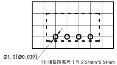
PCB 印刷版图
