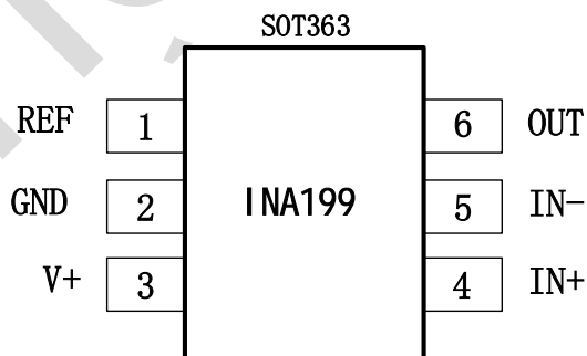
INA199 引脚排列图
