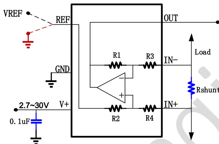
INA199 功能框图
