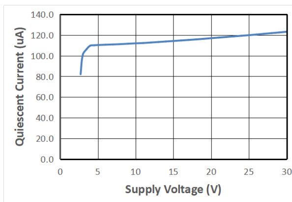
静态电流随电源电压变化
