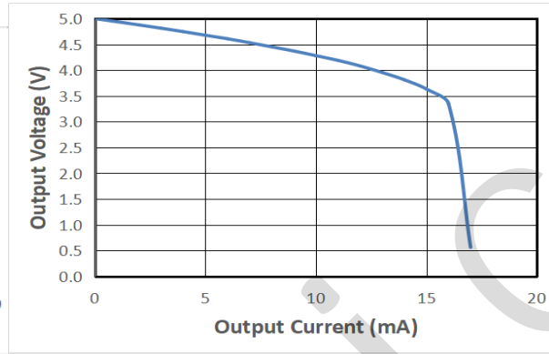
高电平驱动能力
