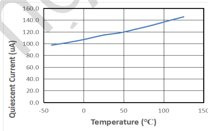
电源电流随温度变化曲线
