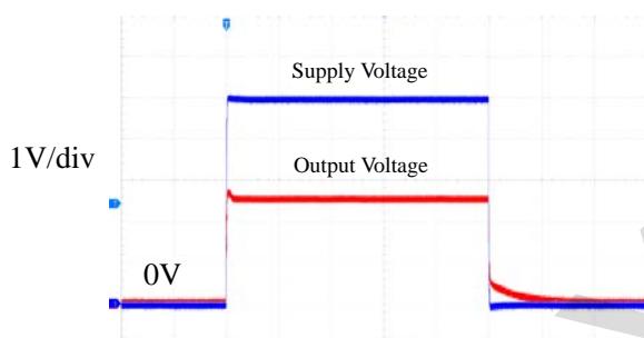
Time(100us/div) 启动响应
