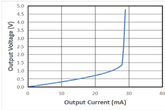
低电平驱动能力
