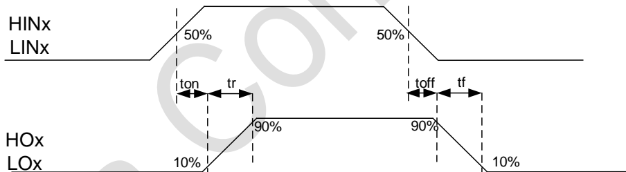
图 5-8 开关时间
