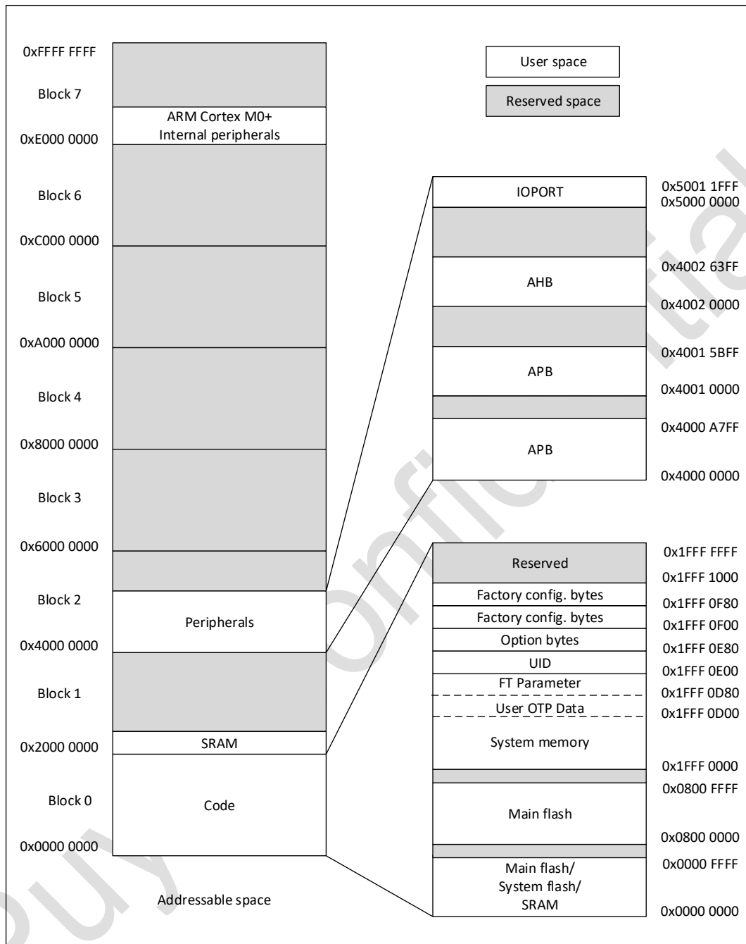
图 4-1 存储器映射
