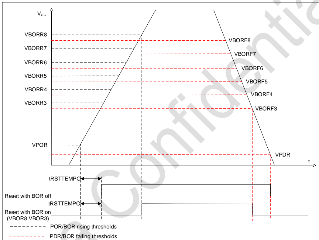
图 2-3 POR/PDR/BOR 阈值
