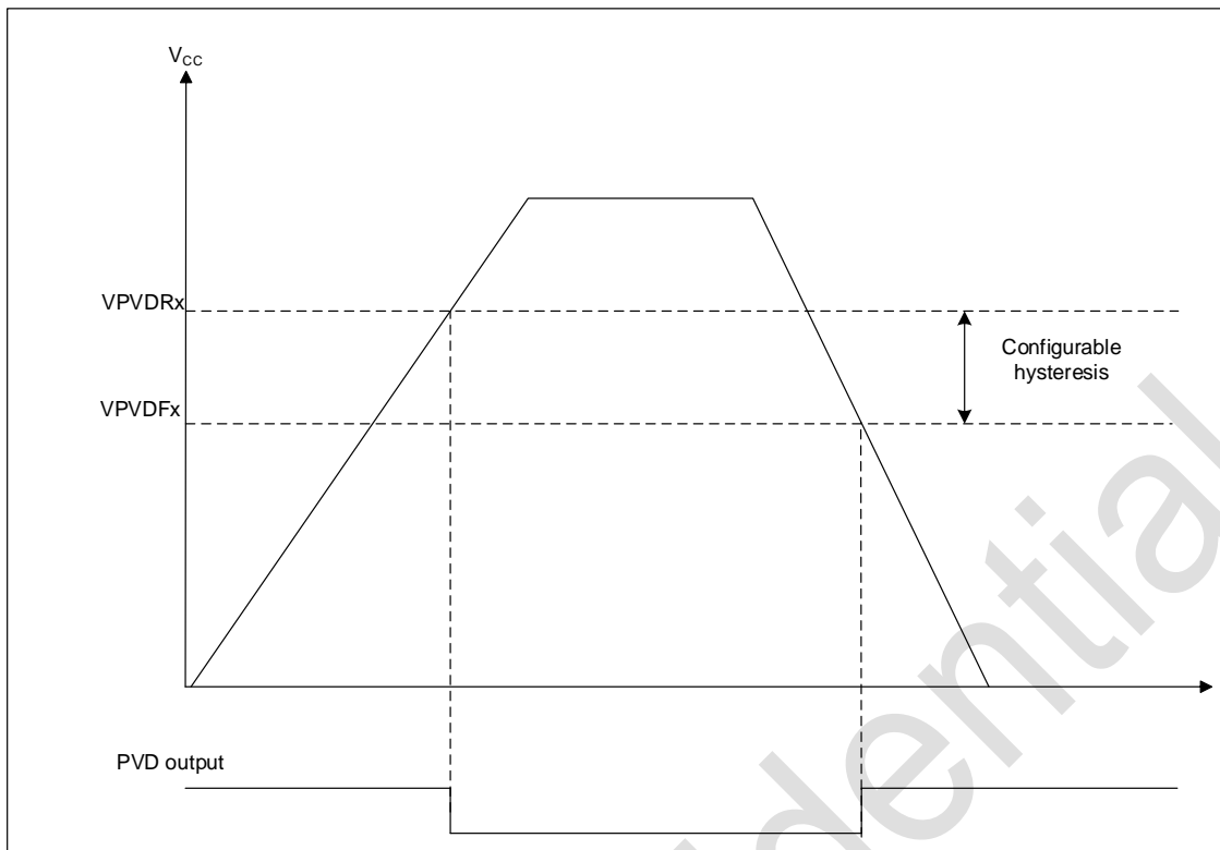
图 2-4 PVD 阈值
