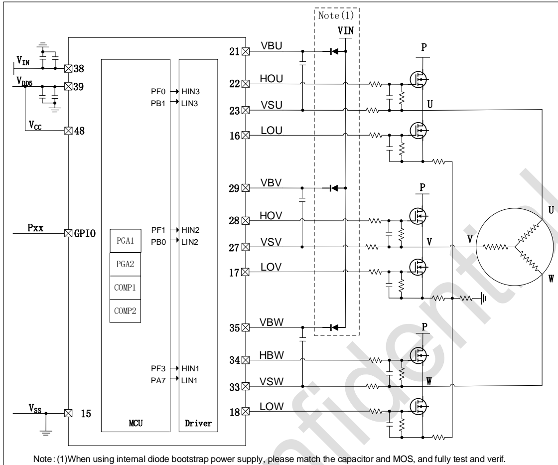
图 6-2 PY32MD540C28T7 推荐应用电路图
