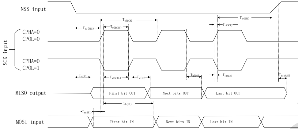
图 5-1 SPI 时序图 – 从机模式, CPHA = 0
