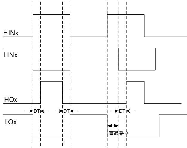
图 5-7 直通保护
