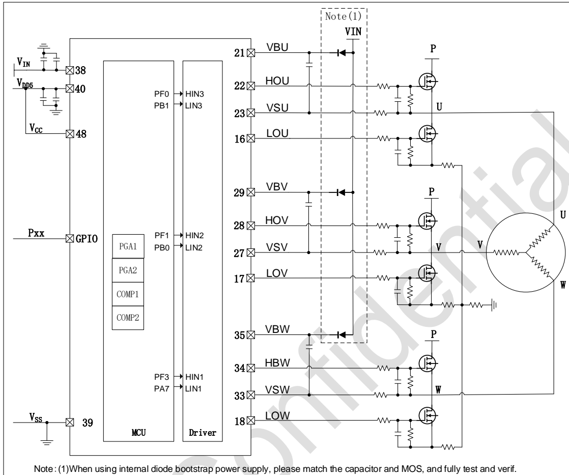
图 6-1 PY32MD540C18T7 推荐应用电路图
