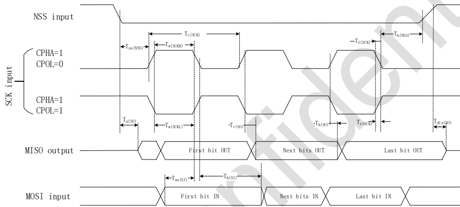
图 5-2 SPI 时序图 – 从机模式, CPHA = 1
