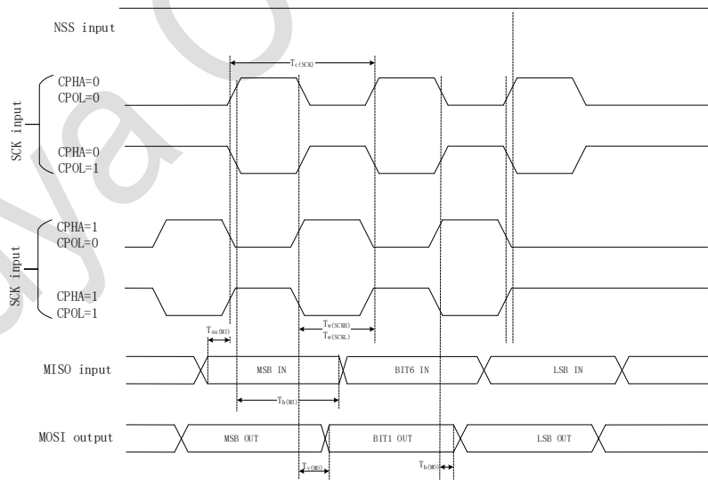
图 5-3 SPI 时序图 – 主机模式
