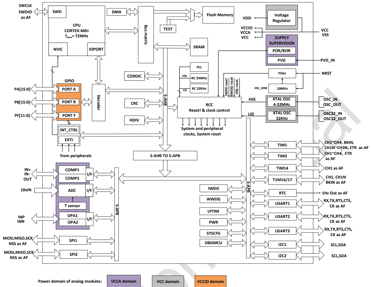
图 1-1 功能模块
