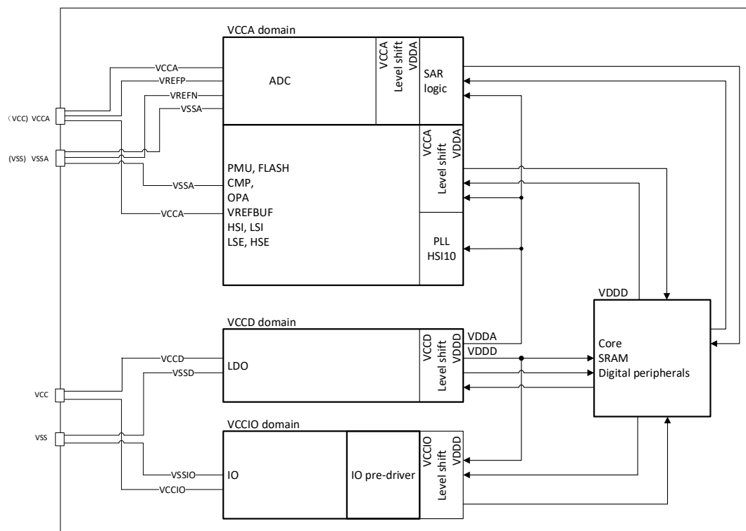
图 2-2 电源框图
